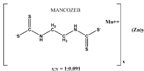
Figura 1. Estructura química del mancozeb.
