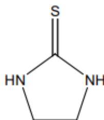
Figura 2. Estructura química de etilentiourea
